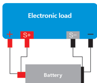
▲ 放电接线图
