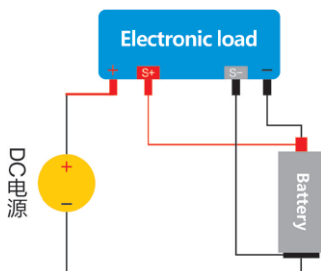
▲ 充电接线图
